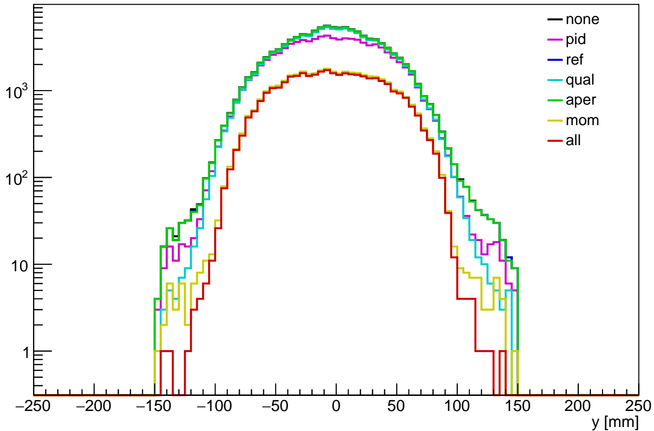
tkd y distribution (recmc)
