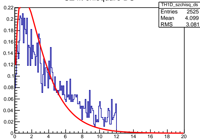
SZ fit chisquare DS
