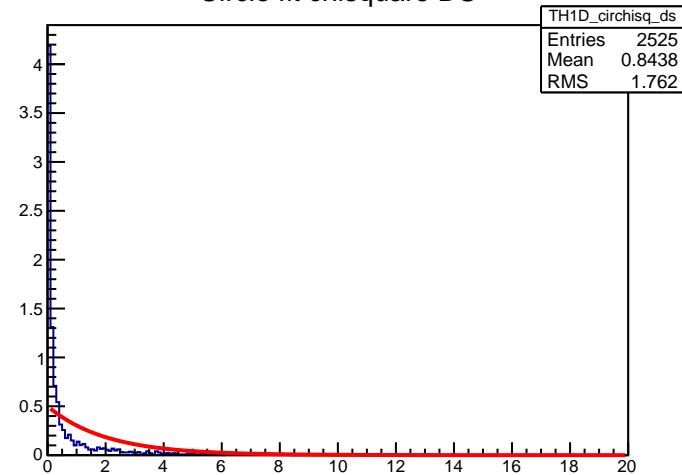
Circle fit chisquare DS
