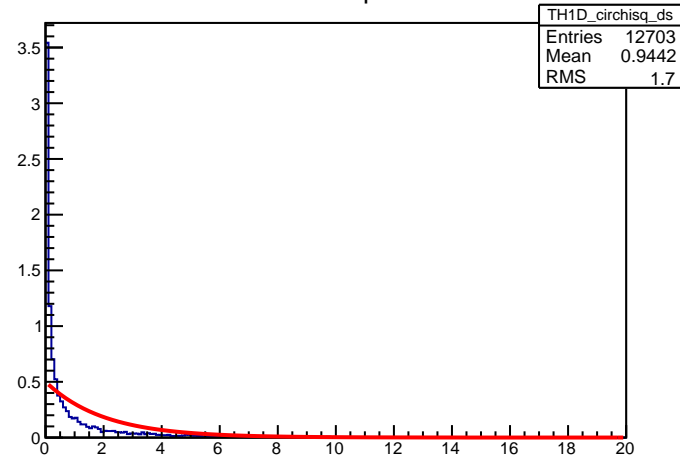
Circle fit chisquare DS
