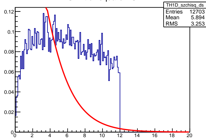
SZ fit chisquare DS
