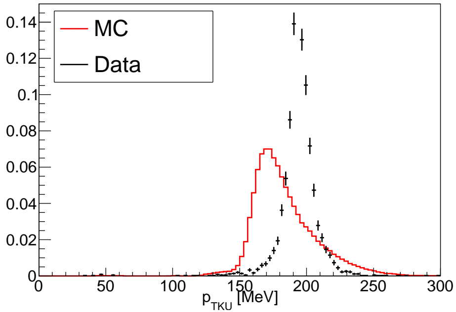
Muon Momentum
