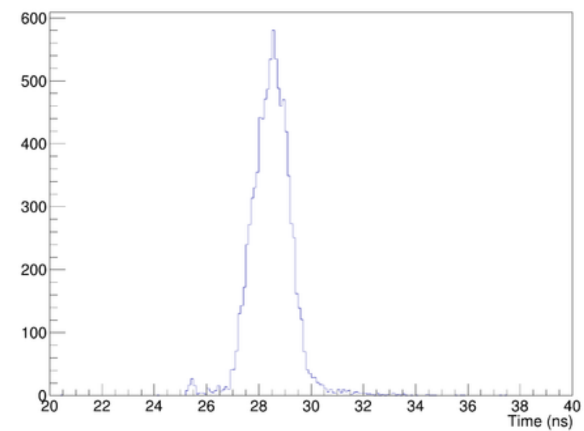
TOF0-&gt;1, Run 7835
