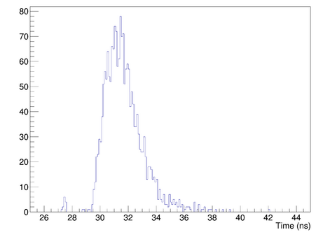
TOF1-&gt;2, Run 7835
