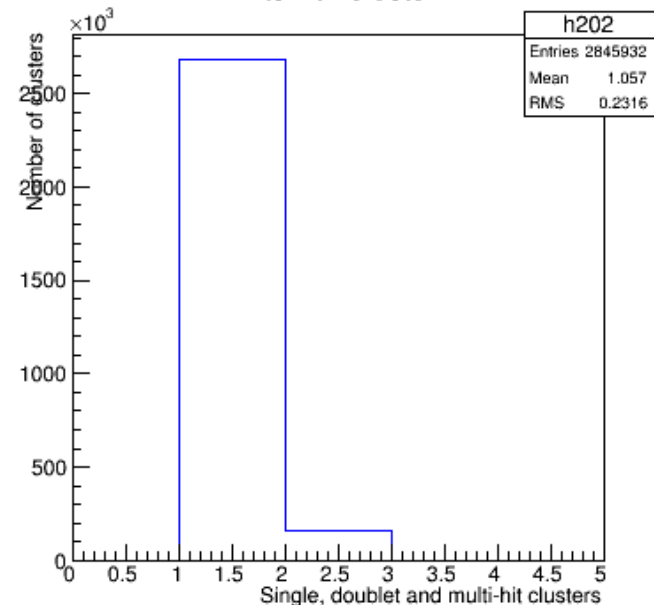
Hits Per Cluster
