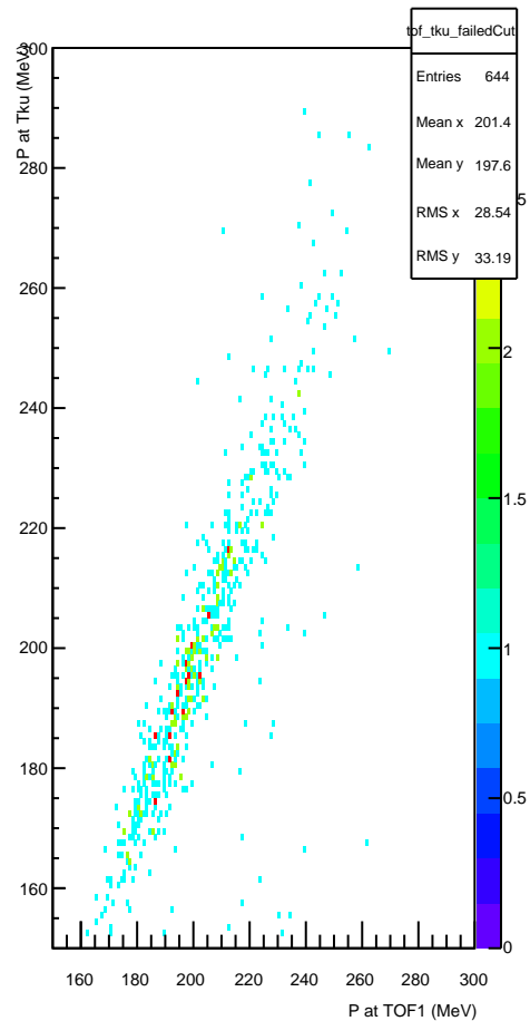
TOF P vs Tku P (P-values &lt; 0.05)
