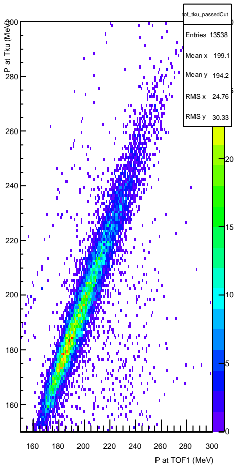
TOF P vs Tku P (P-values &gt; 0.05)
