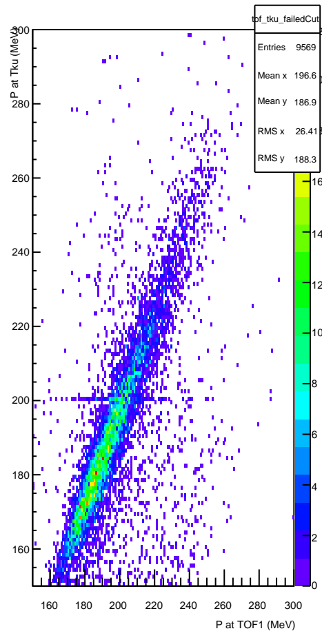
TOF P vs Tku P (P-values &lt; 0.05)
