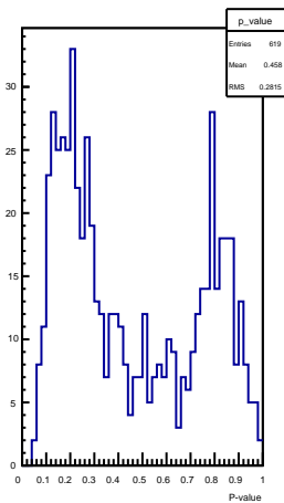
P-value
