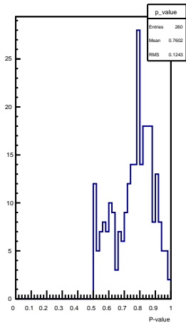
P-value
