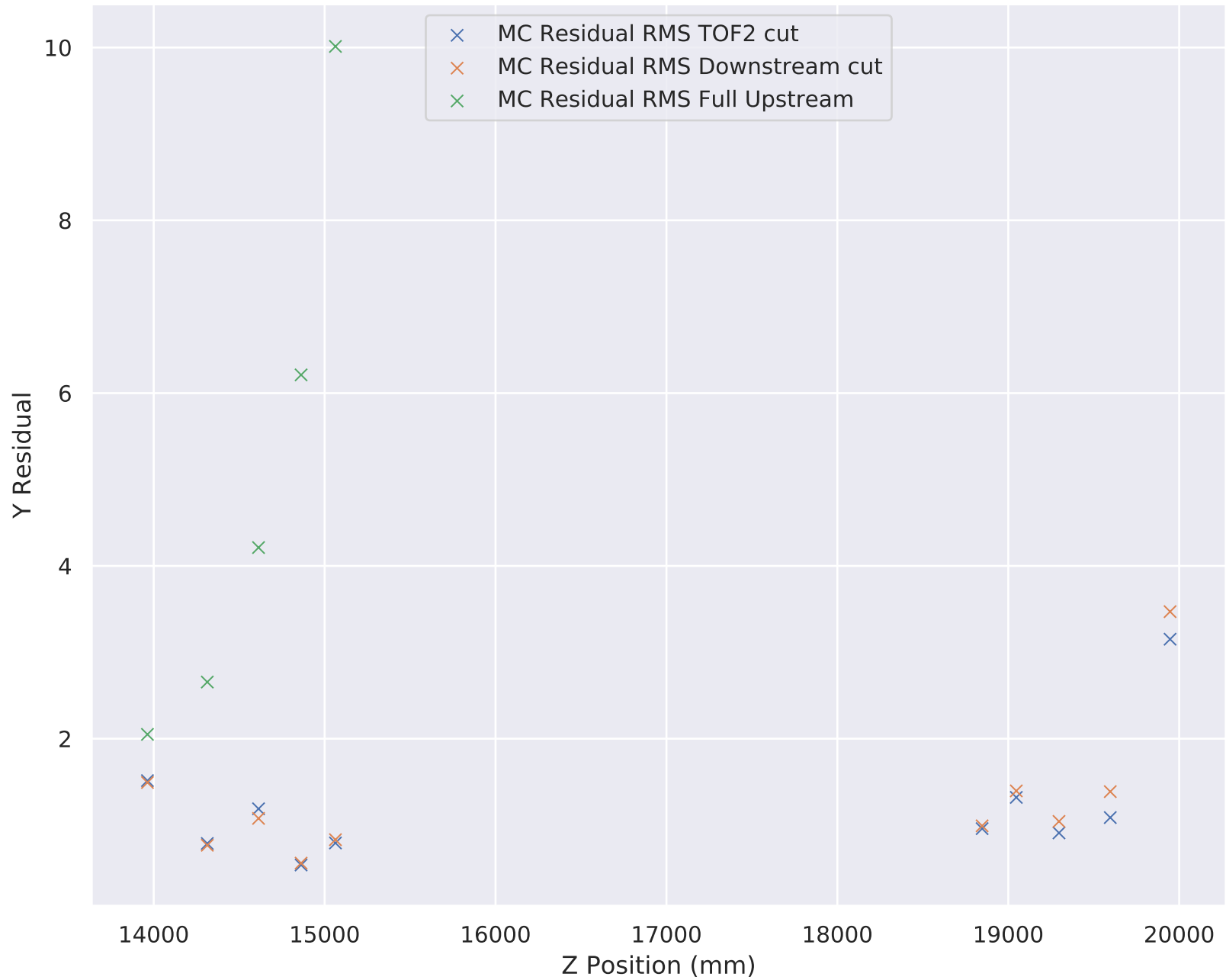
6-140 Wedge Solenoid Y Residual RMS
