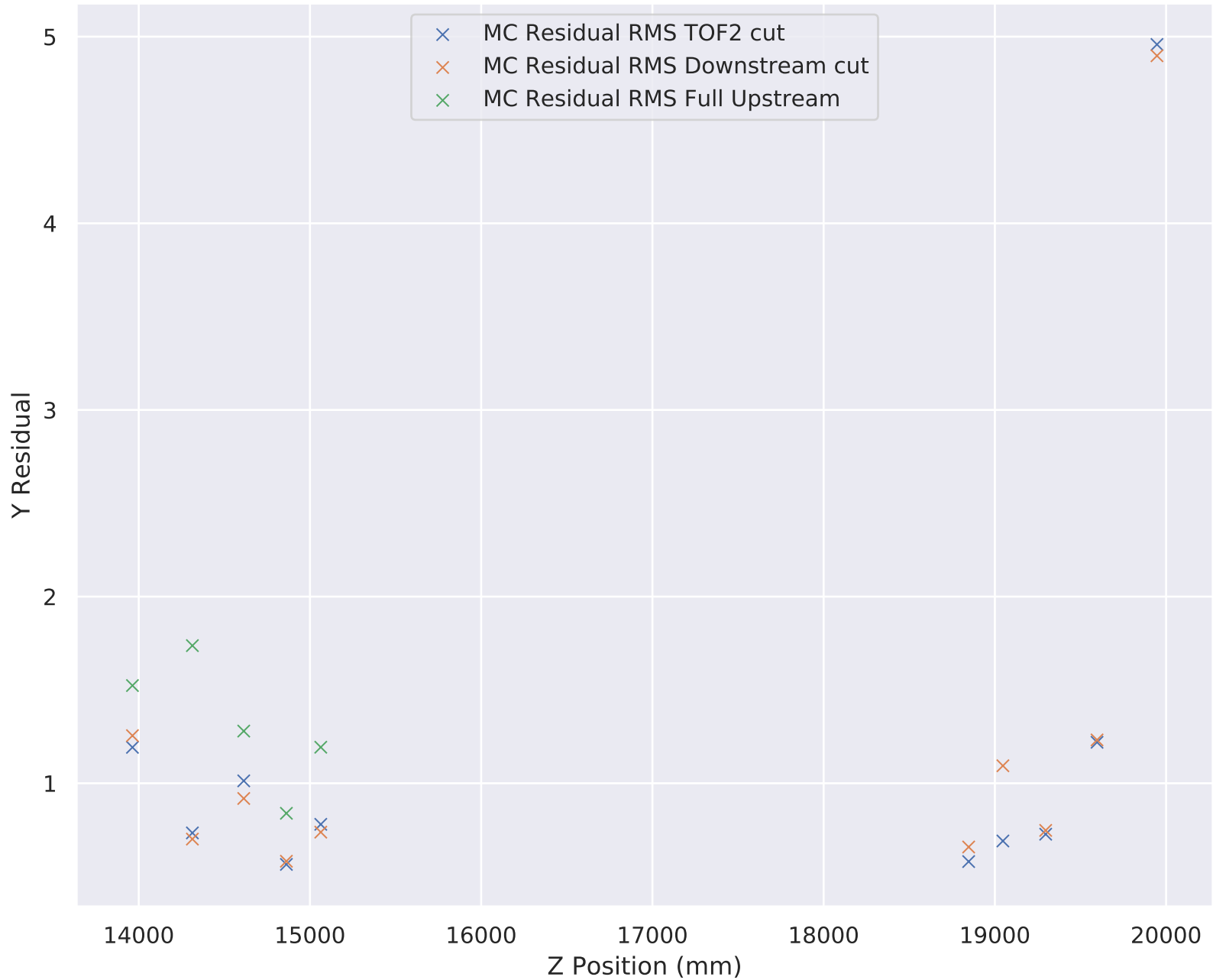
6-140 Wedge Solenoid Y Residual RMS
